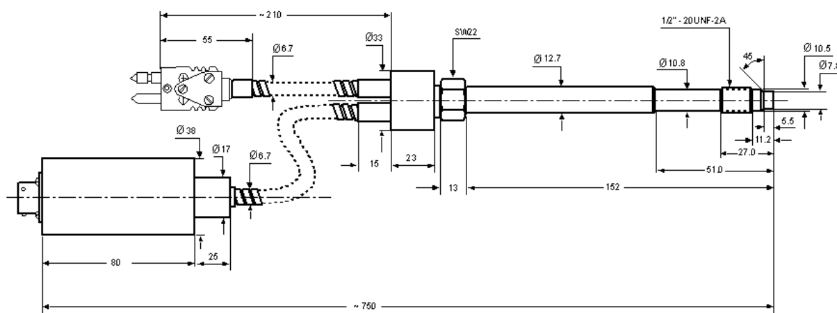
Wymiary przetwornika ciśnienia PC-38K-CT
