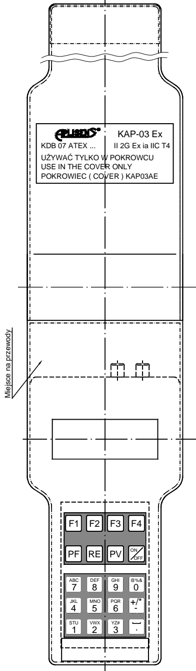
Rys.2 Pokrowiec komunikatora KAP-03Ex
