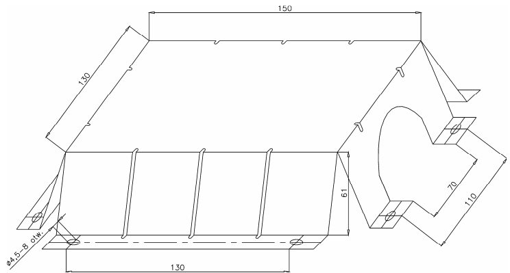
Rys.1 Plomba pływaka
